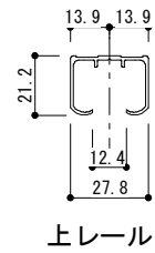
上レール
