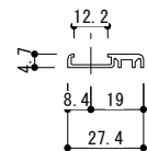
下レール
